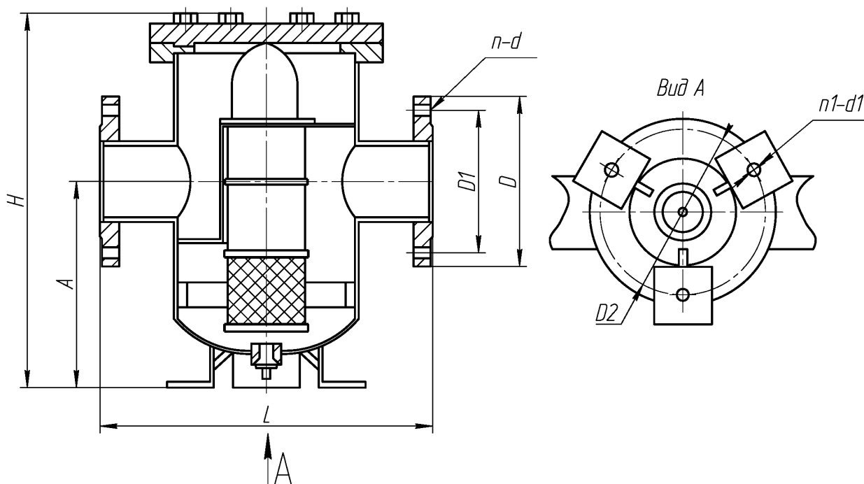
Рисунок А2 Фильтр Dn 50-150
