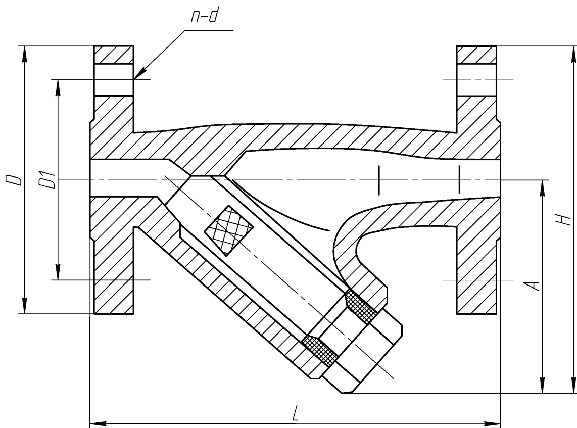
Рисунок А1 Фильтр Dn 25-50
